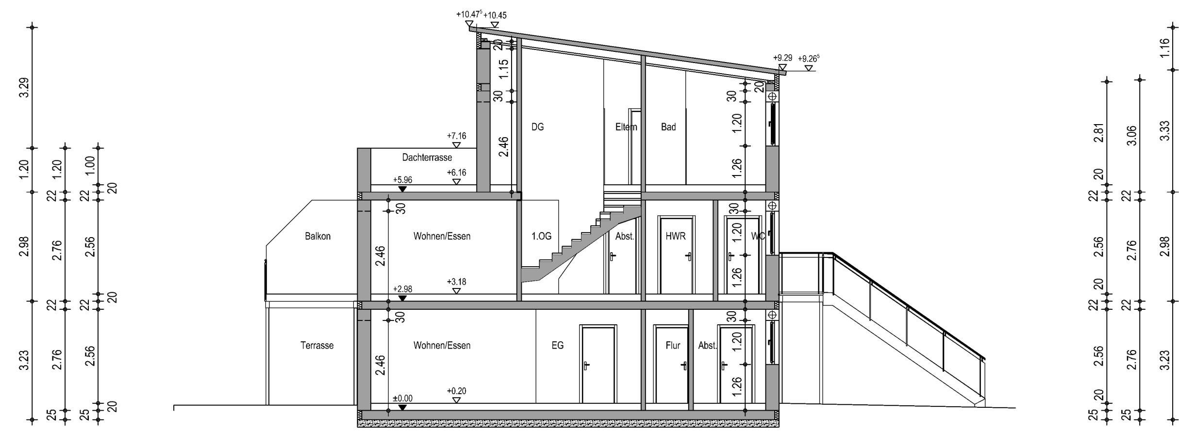
Schnitt M 1:100
